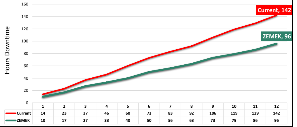
DOWNTIME PER DRAGLINE
